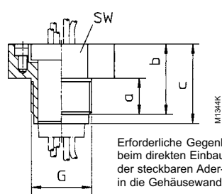
Steckbare Aderleitungsdurchführungen, 8174/2
