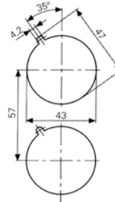
Ansicht ohne Klappdeckel View without hinged cover
